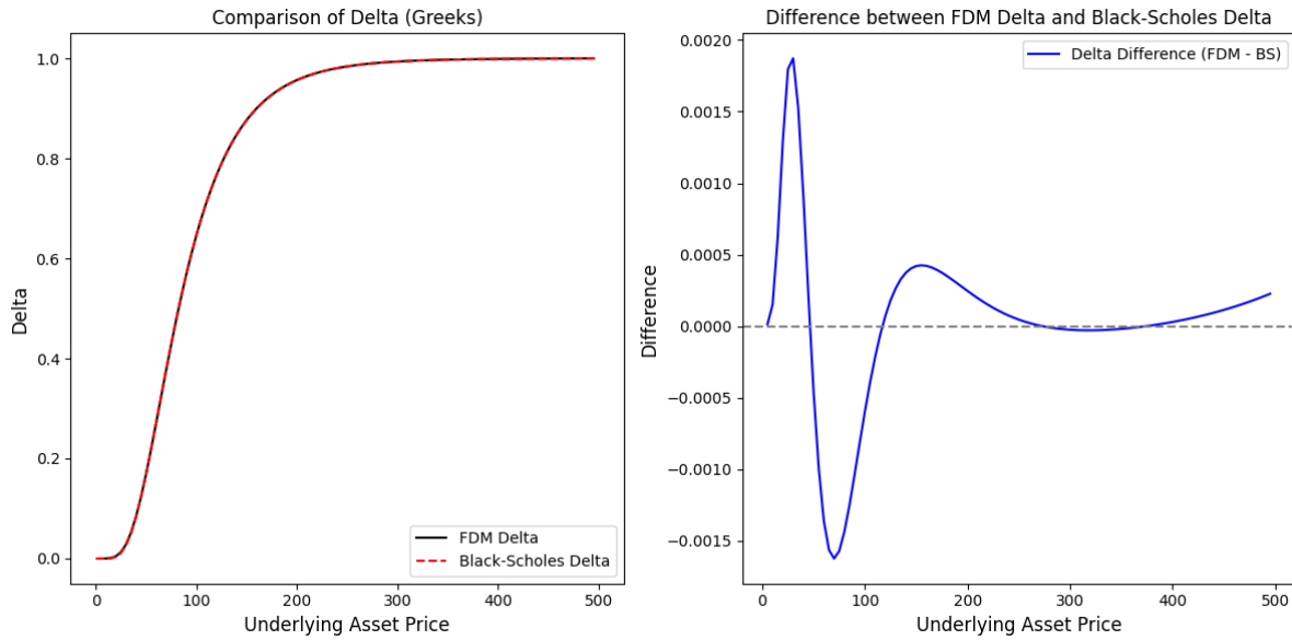
Figure 9. Neumann 경계조건
